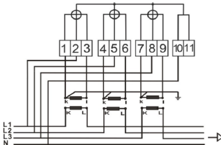
Šema poluindirektnog vezivanja trofaznog električnog brojila na niskonaponsku mrežu
