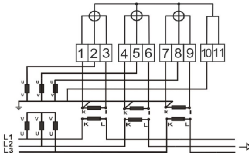
Šema indirektnog vezivanja trofaznog električnog brojila na mrežu
