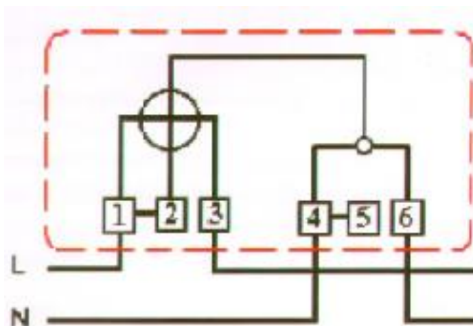
Šema vezivanja monofaznog indukcionog brojila na mrežu niskog napona
